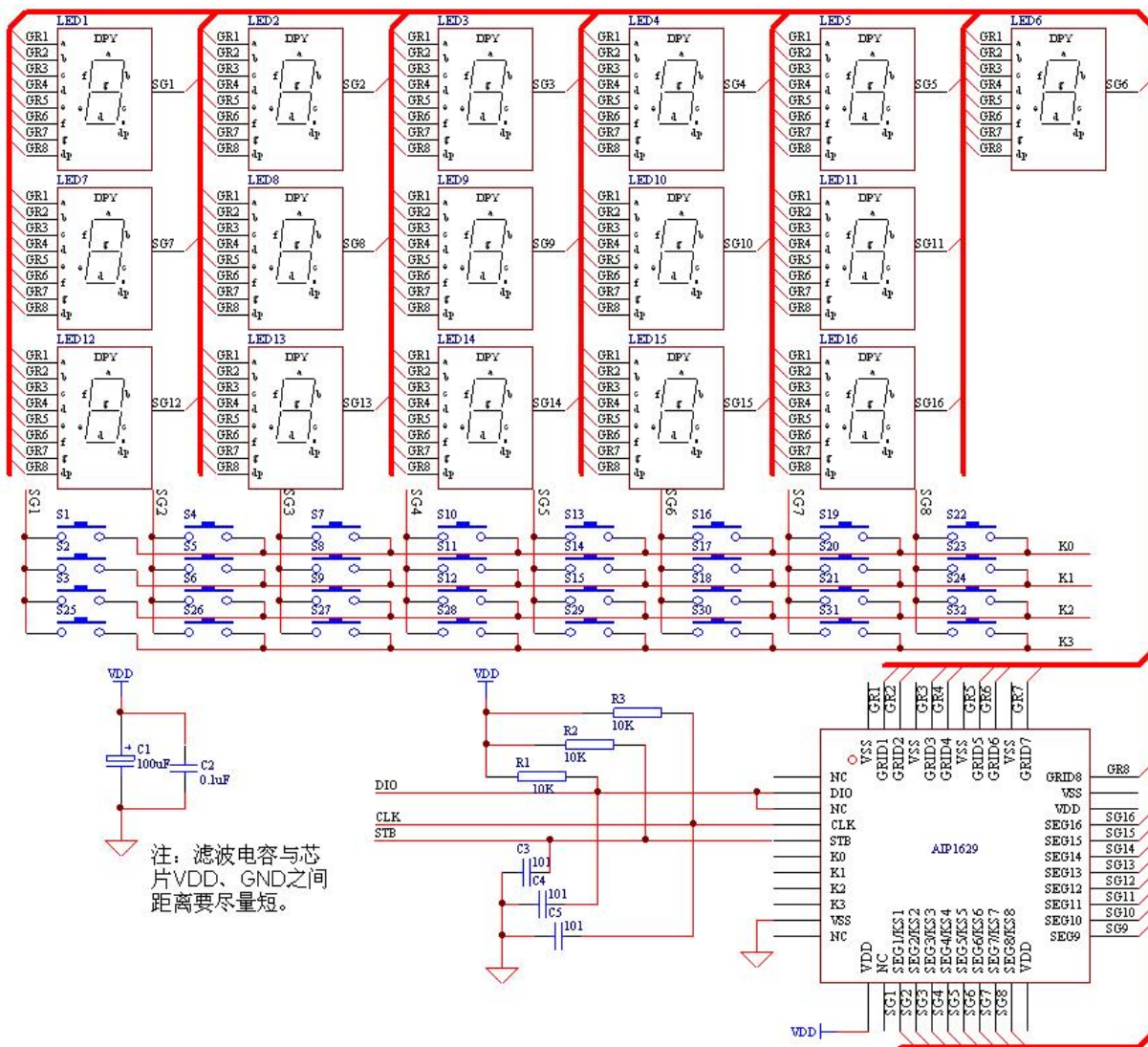
图 17、共阳数码屏应用线路
