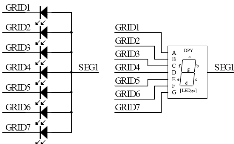
图9、共阳数码管
