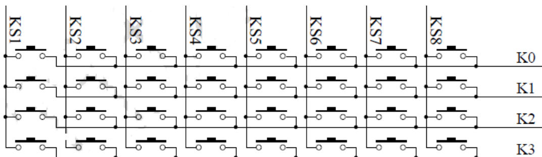
图 4、键扫矩阵
