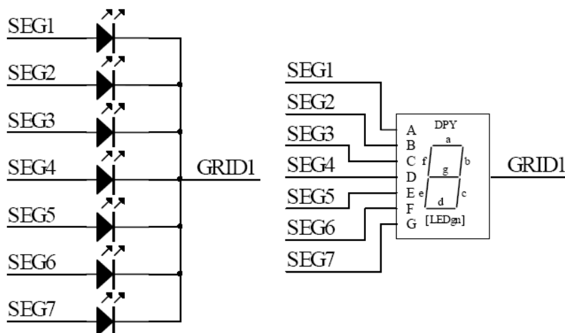
图8、共阴数码管
