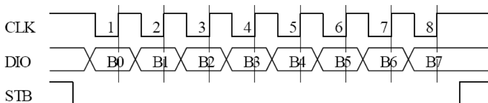
图6、数据接收
