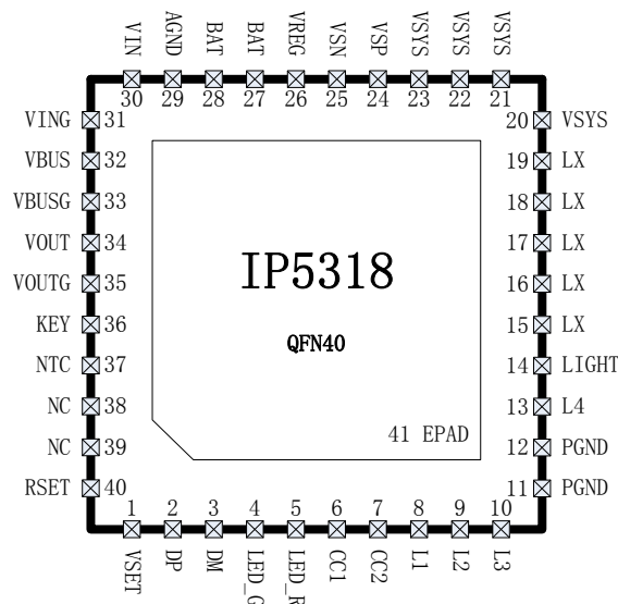
图 3 IP5318/IP5318Q 引脚图
