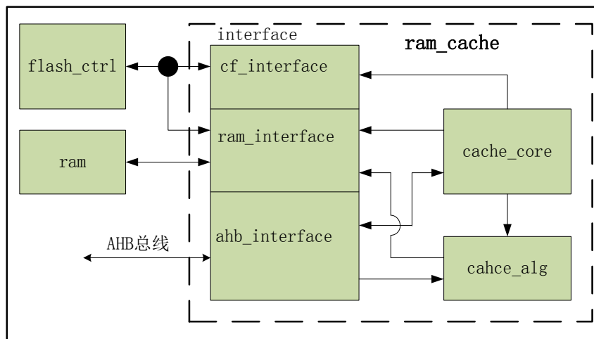
图 6-50 CACHE 内部结构示意图
