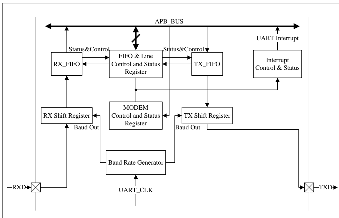
图 6-18 UART 结构图
