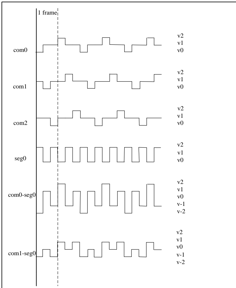
图 6-49 SLCD 驱动波形 1/3duty&1/2bias
