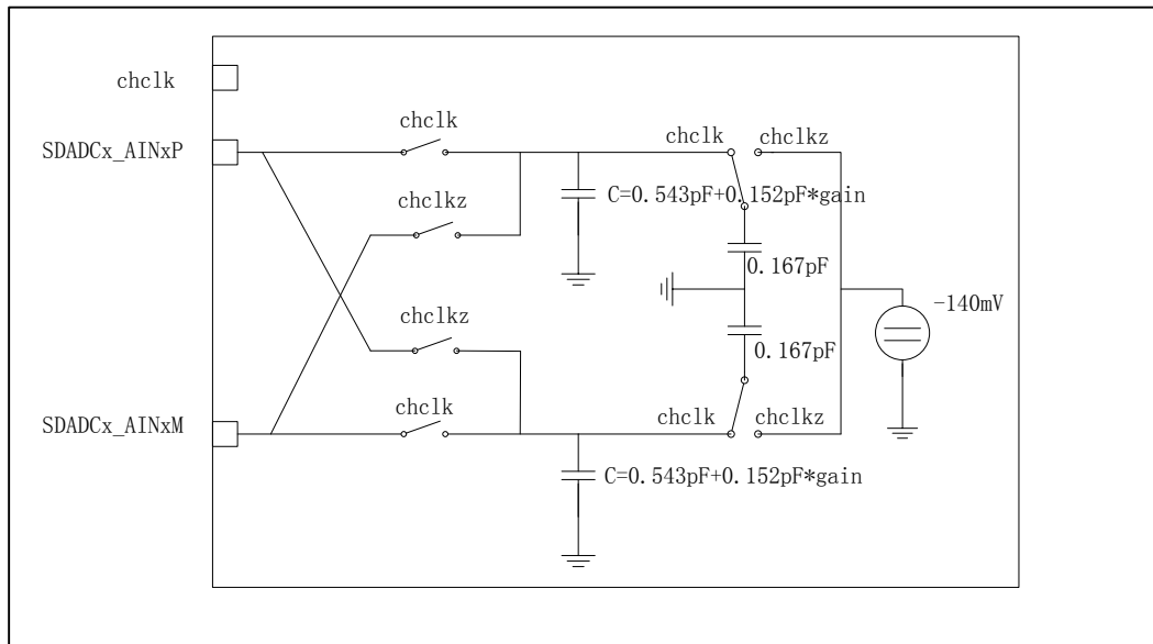
图 6-44 输入阻抗示意图
