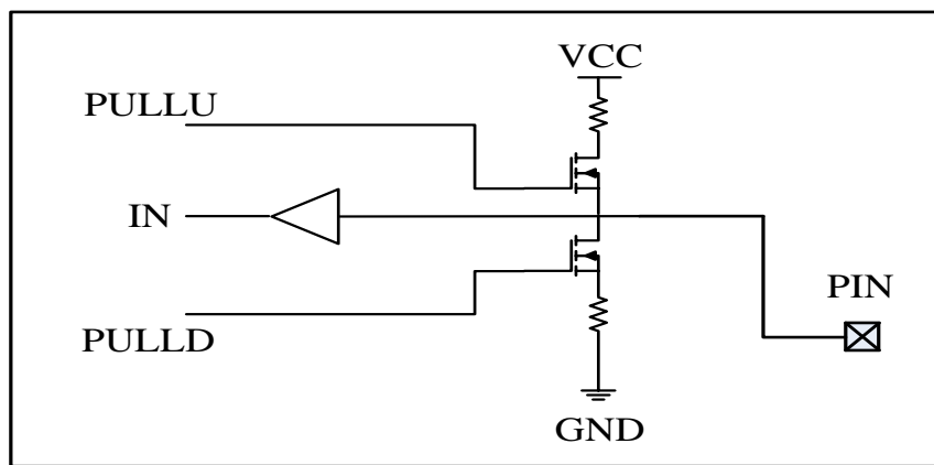
图 6-7 IO 输入上拉下拉
