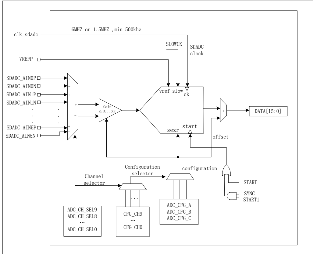
图 6-40 内部结构示意图
