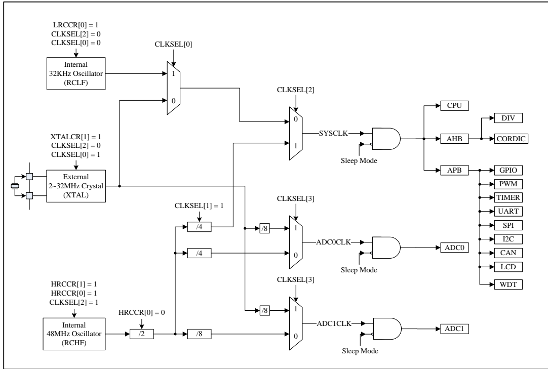
图 6-1 时钟连接图
