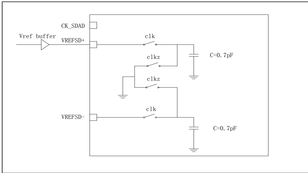
图 6-45REFP 阻抗示意图
