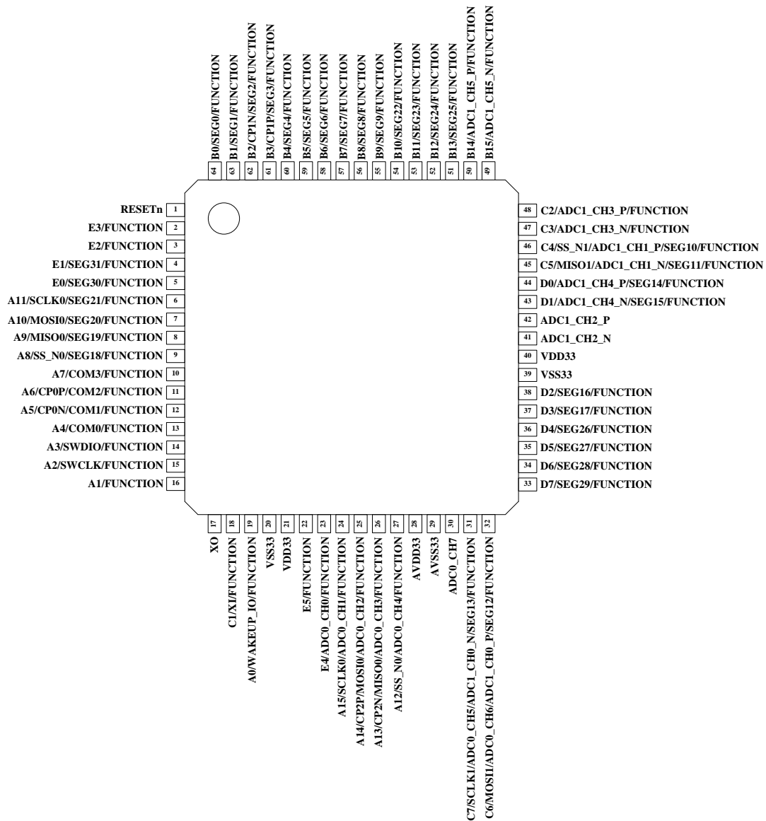
图 5-4 RCT6 封装管脚配置图
