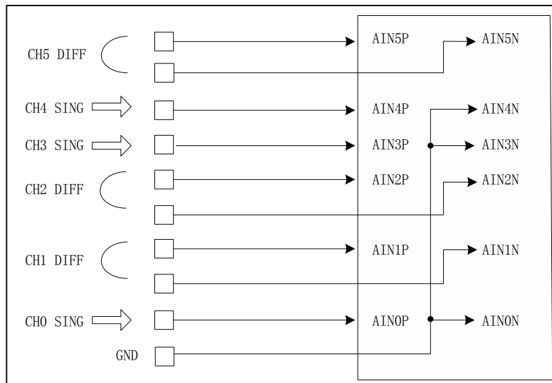
图 6-43 混合模式配置示意图
