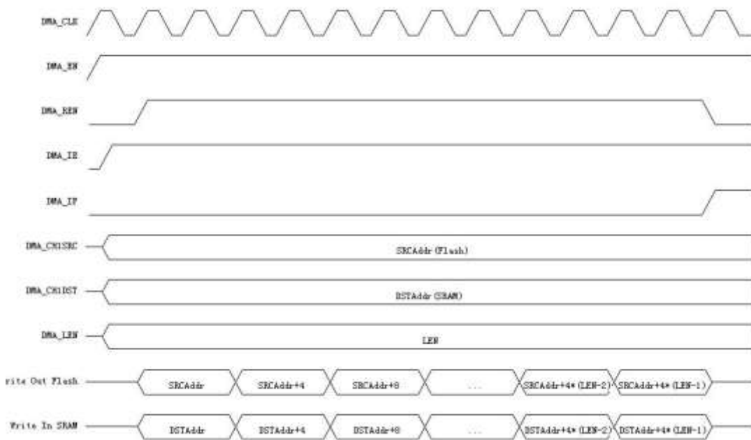
图 6-46 Flash 内数据写入到内存
