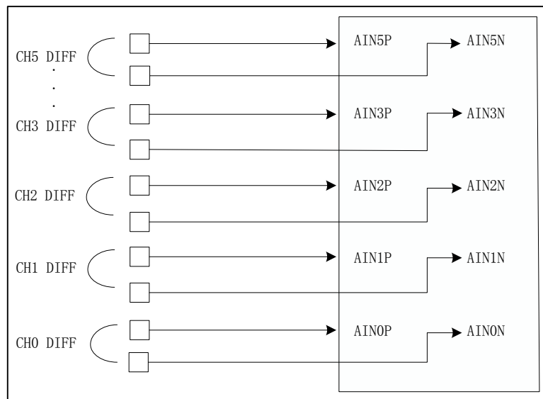
图 6-41 差分输入管脚配置示意图
