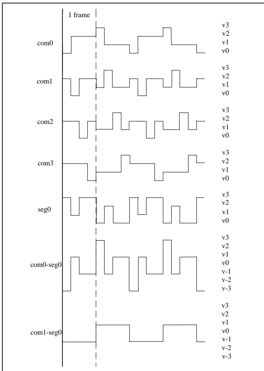
图 6-48 SLCD 驱动波形 1/4duty&1/3bias
