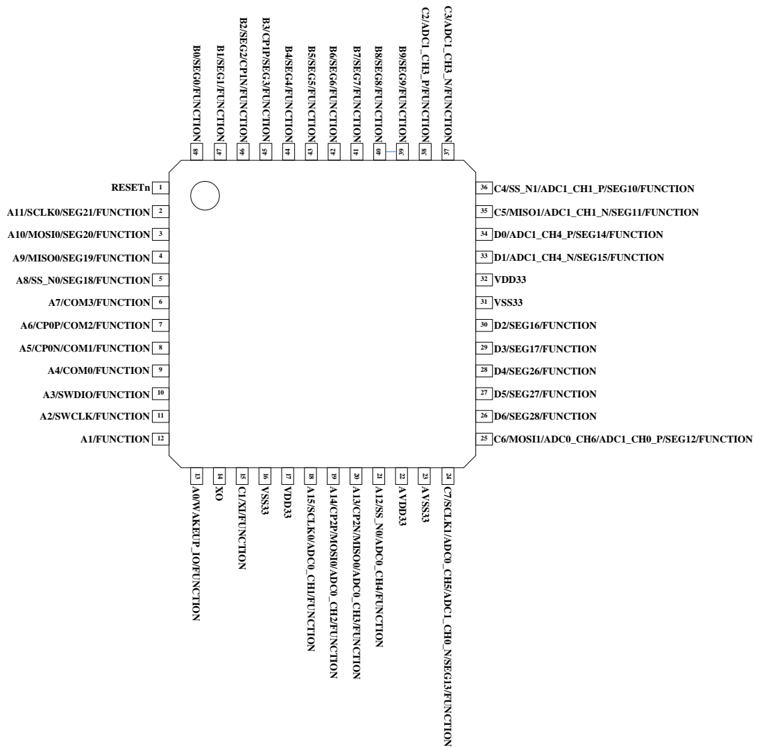
图 5-2 CBT6 封装管脚配置
