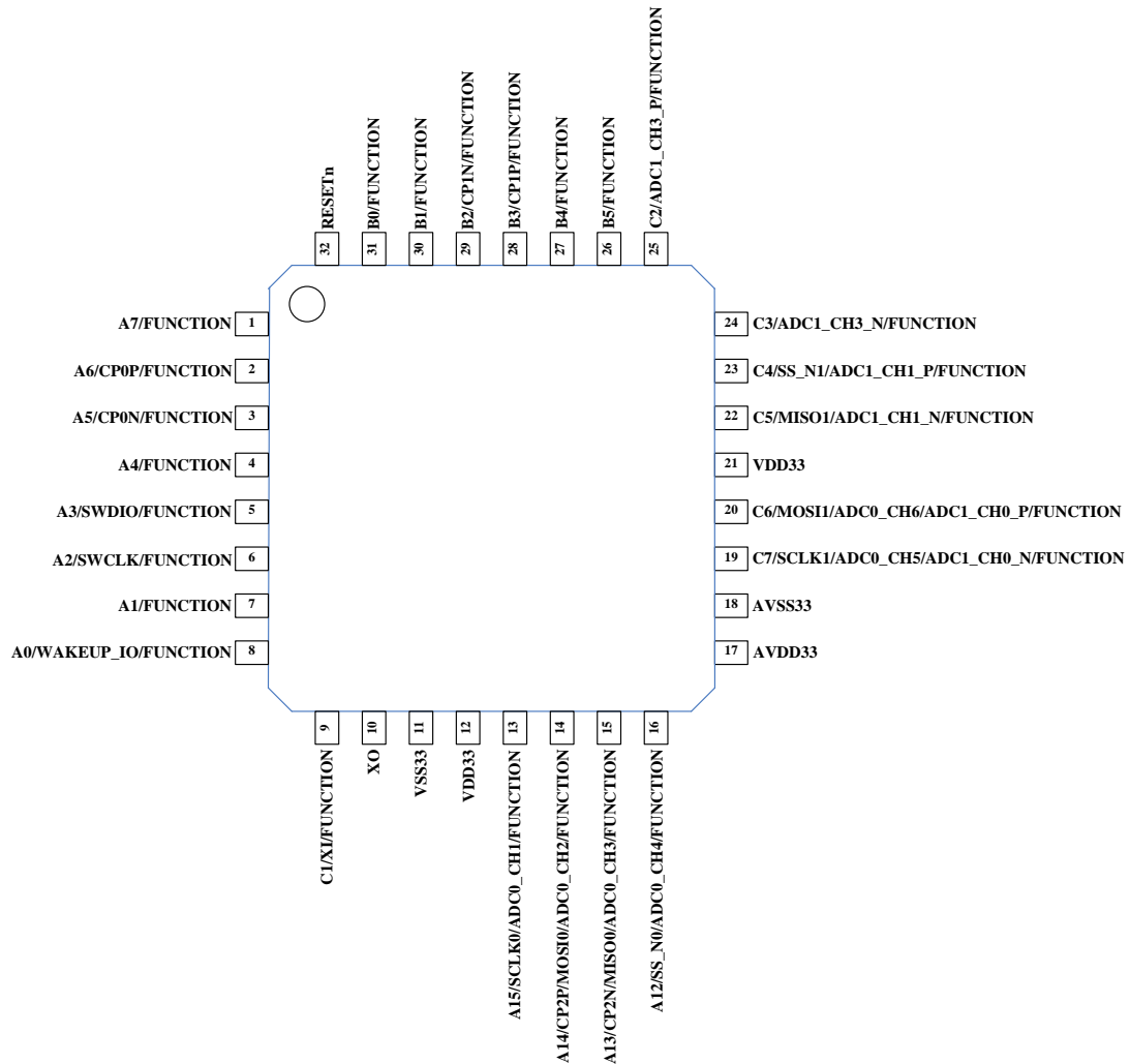
图 5-1 KCT6 封装管脚配置
