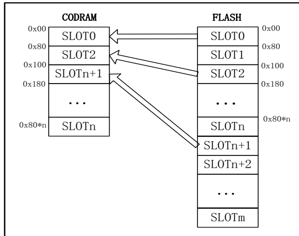
图 6-51 内部 RAM 与外部 FLASH SLOT 对应图
