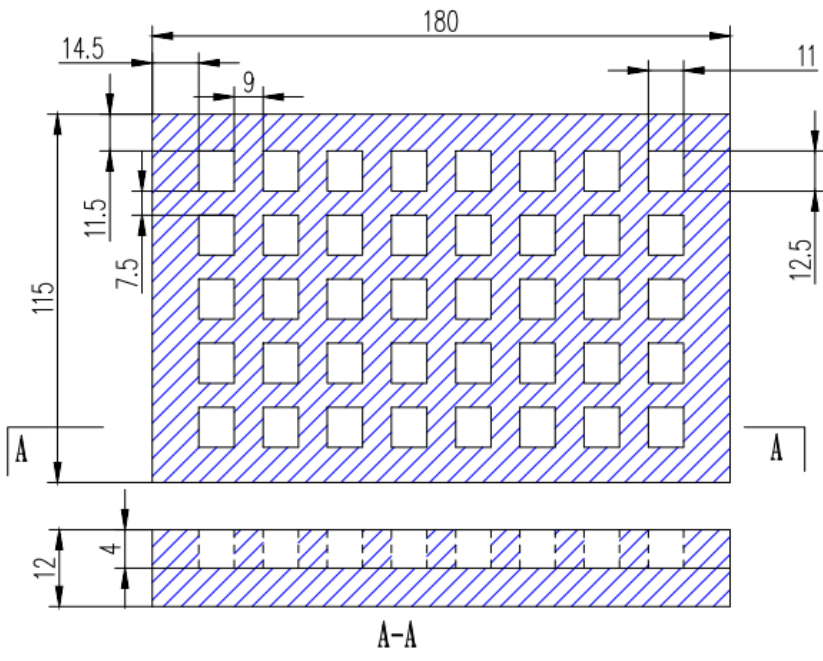
S,T 壳包装盘
