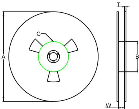
轮盘尺寸图
