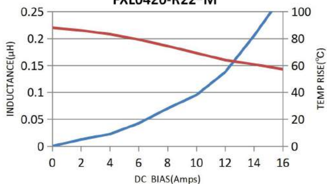
FXL0420-R22-M
