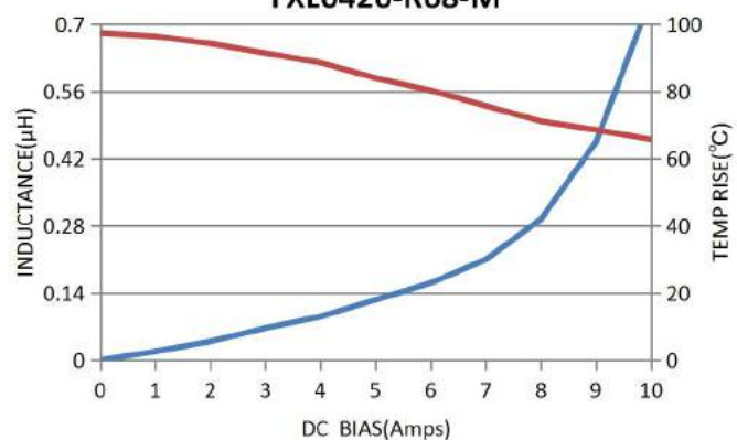
FXL0420-R68-M
