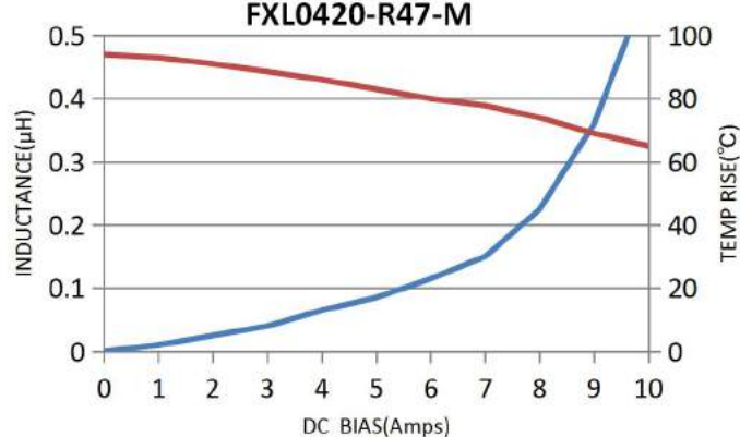
FXL0420-R47-M
