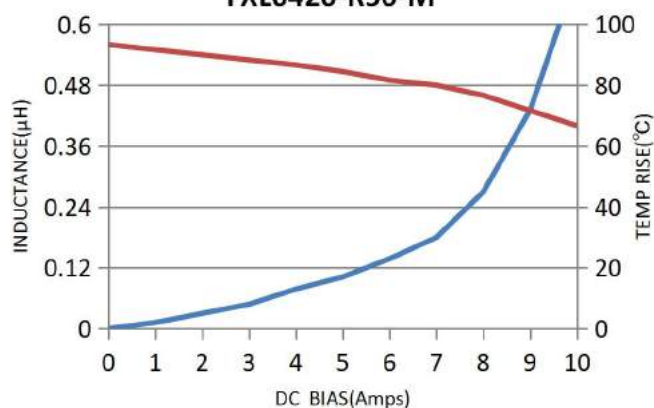
FXL0420-R56-M
