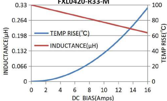
FXL0420-R33-M
