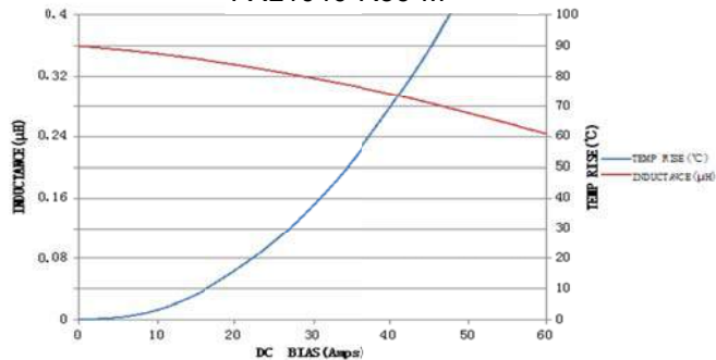
FXL1040-R36-M
